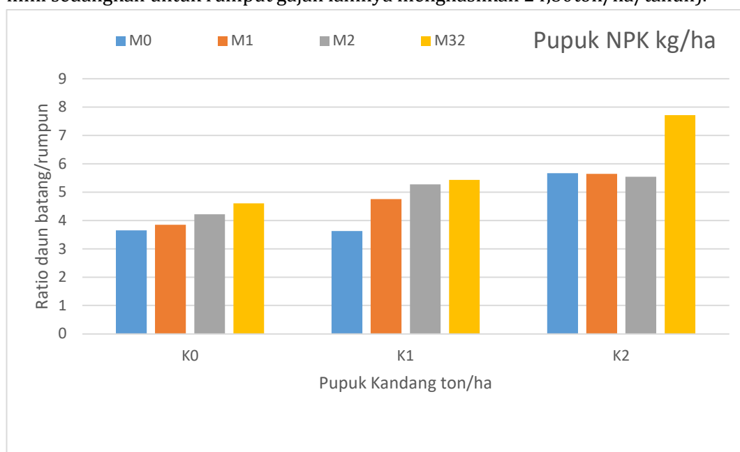
Gambar 4. Diagram kombinasi pupuk kandang dan NPK terhadap ratio daun batang.
