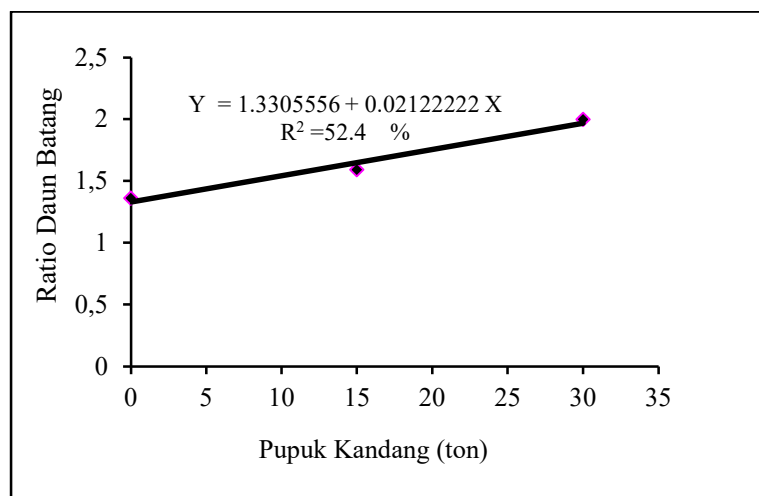
Gambar 5. Grafik hubungan antara dosis pupuk kandang dengan ratio daun batang rumput gajah mini.
