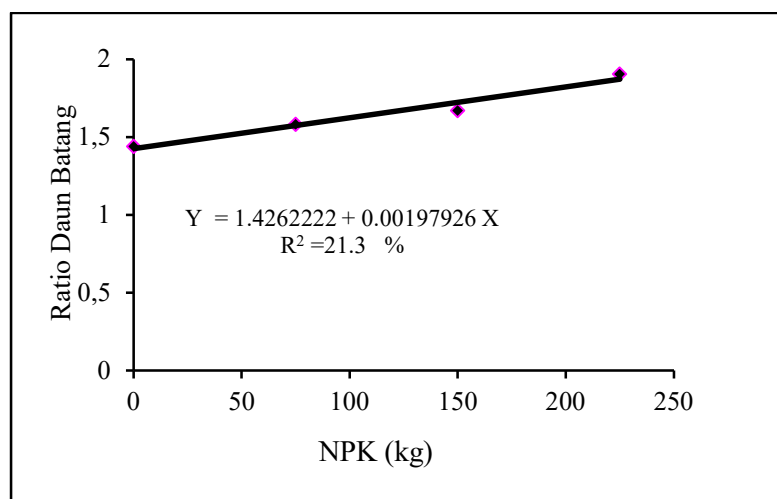
Gambar 6. Grafik hubungan antara dosis pupuk NPK dengan ratio daun batang gajah mini.
