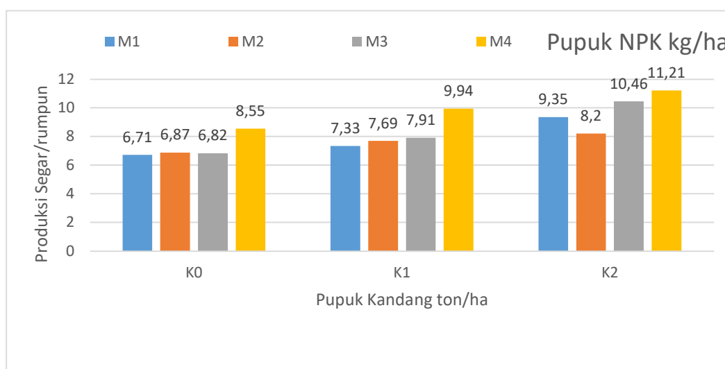
Gambar 1. Diagram kombinasi pupuk kandang dan NPK terhadap produksi segar.
