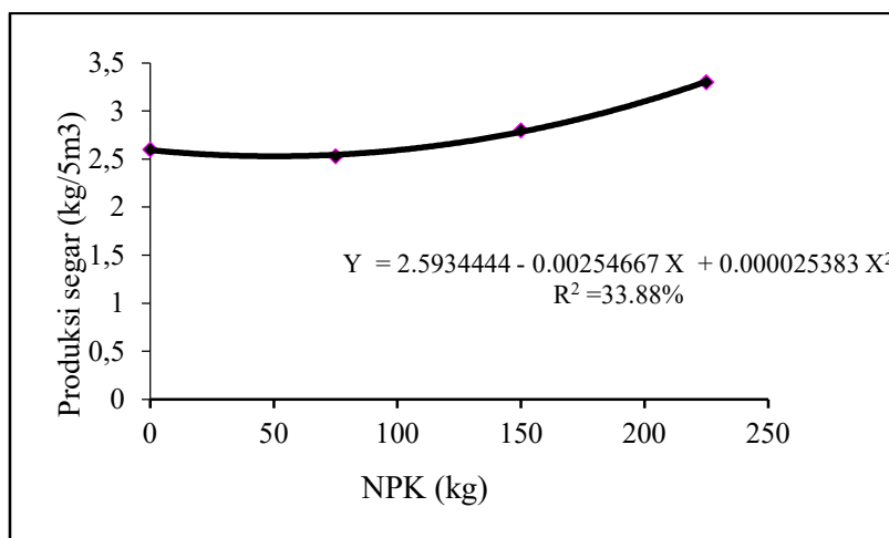
Gambar 3. Grafik hubungan antara dosis pupuk NPK dengan produksi segar rumput gajah mini.
